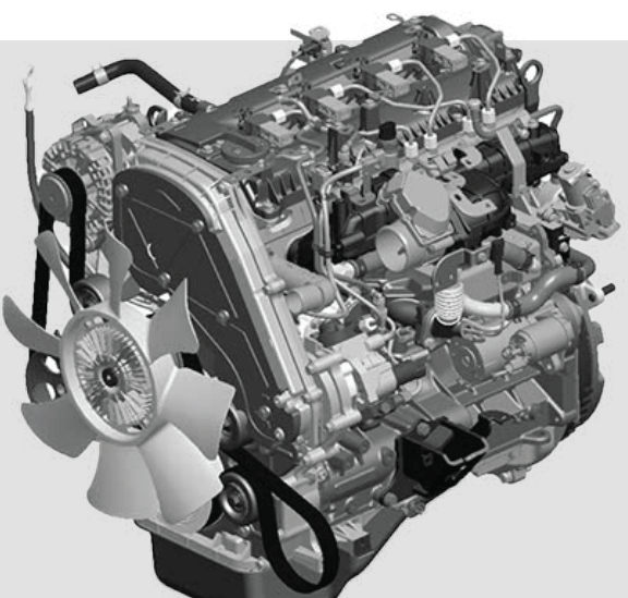
Động cơ D4CB Động cơ đạt công suất tối đa 100 kW tại 3.800 vòng/phút và mô-men xoắn cực đại 294 N.m tại 1.250-3.000 vòng/phút.
